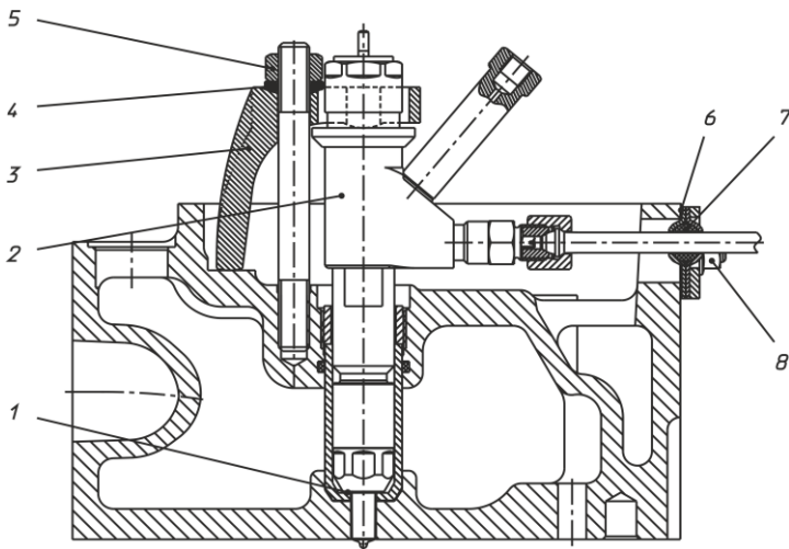
Рисунок 13а – Установка форсунки в головке цилиндров: 1 – шайба 312471-П34; 2 – форсунка; 3 – скоба крепления форсунки; 4 – шайба 312466-П2; 5 – гайка М12×1,25-6Н; 6 – прокладка переходника; 7 – уплотнитель; 8 – гайка с фланцем М8×1,25-6Н
