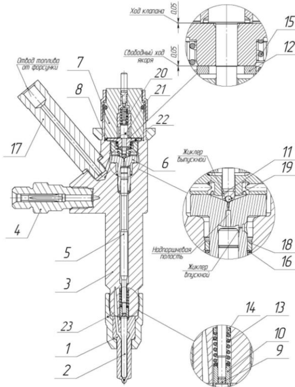
Рисунок 13 – Форсунка:
